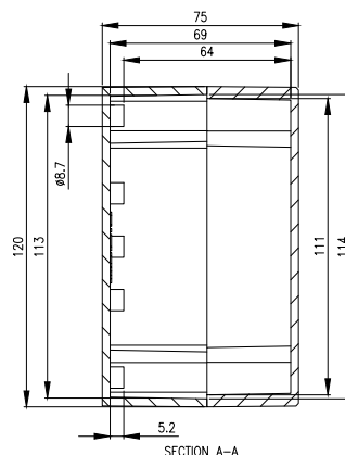
SECTION A-A
