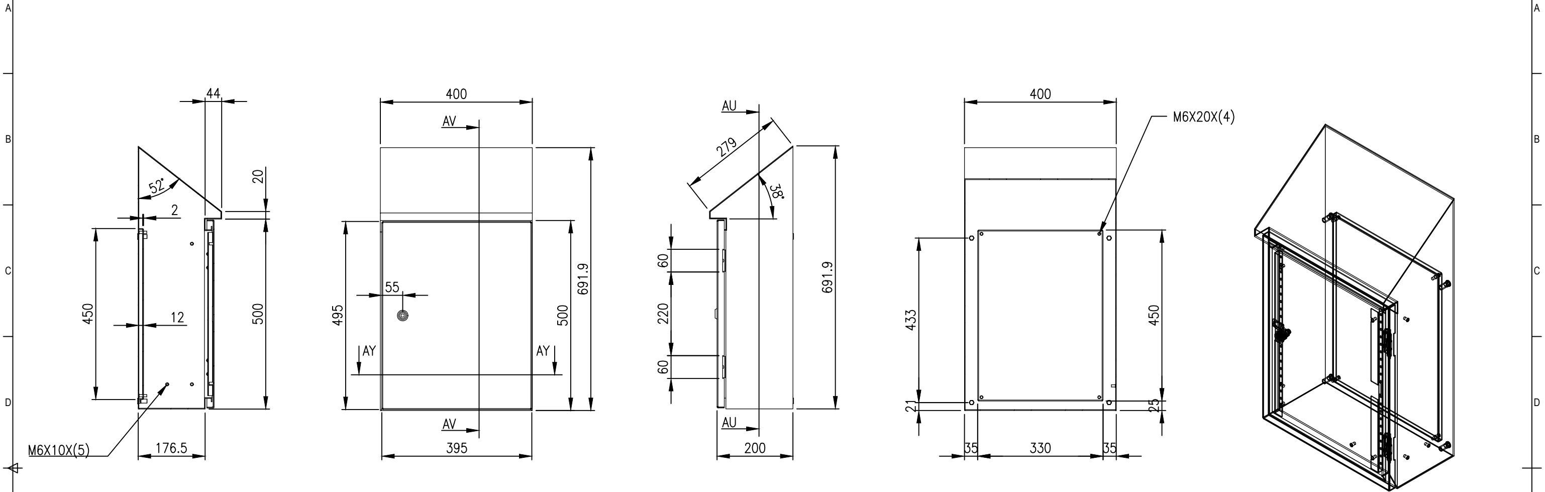
SECTION AV-AV
