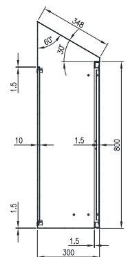
SECTION AV-AV
