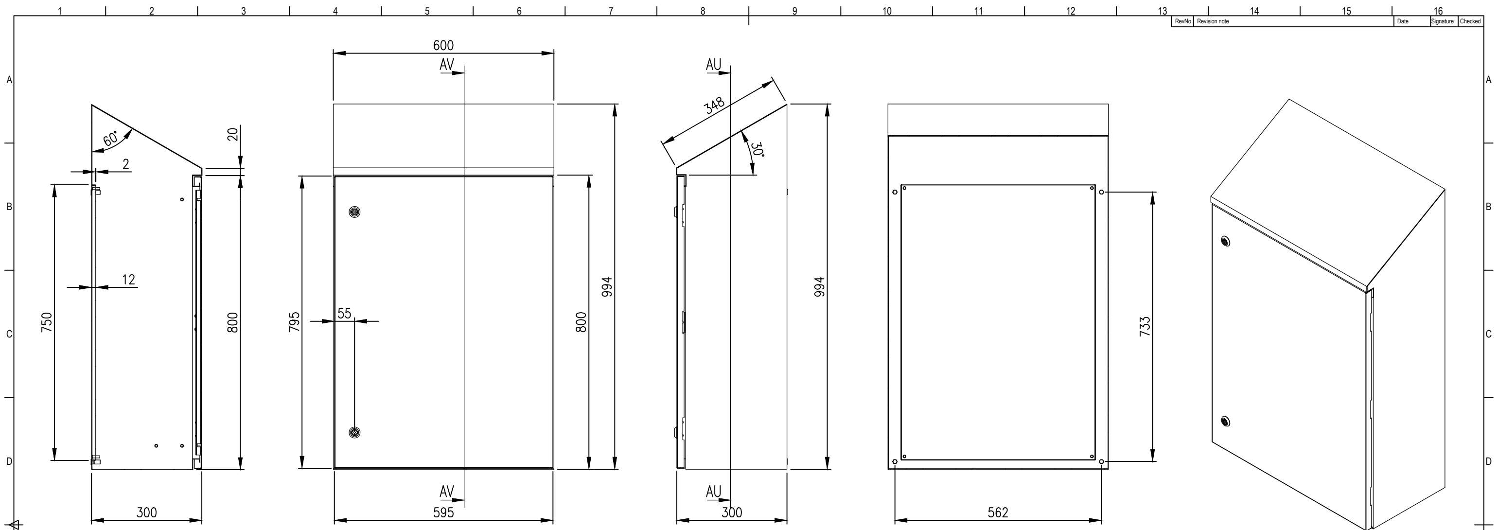
SECTION AV-AV
