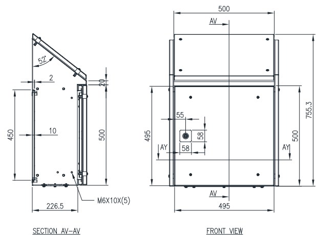
SECTION AV-AV
