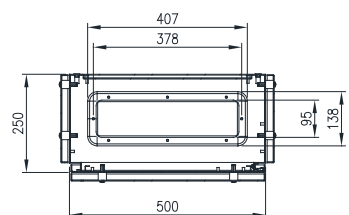
SECTION AY-AY
