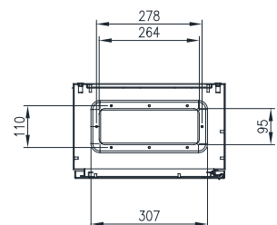
SECTION AY-AY
