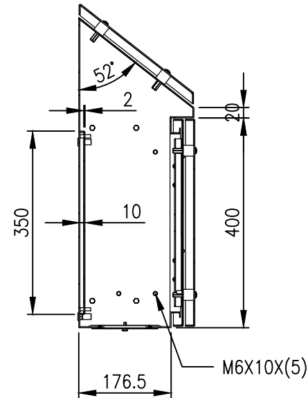
SECTION AV-AV
