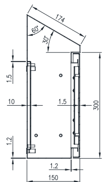
SECTION AV-AV
