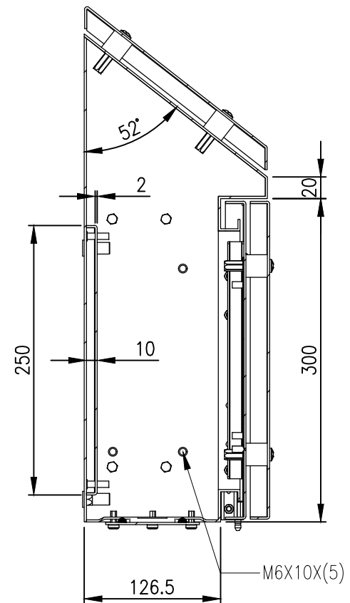
SECTION AV-AV
