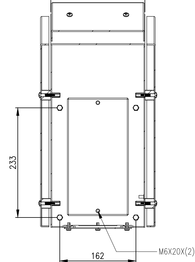
SECTION AU-AU
