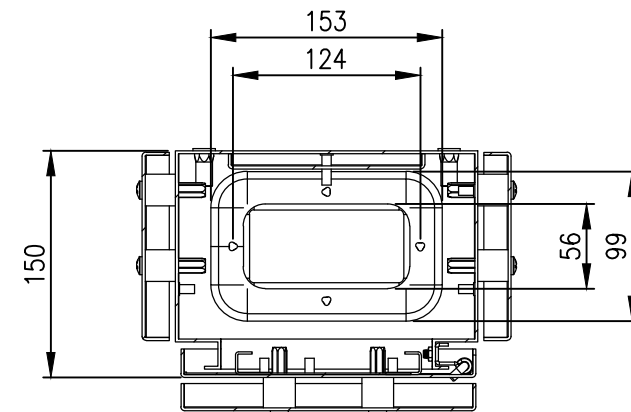
SECTION AY-AY
