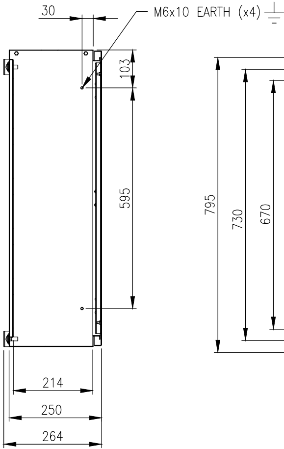
SECTION AY-AY
