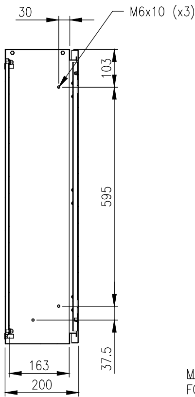
SECTION AY-AY
