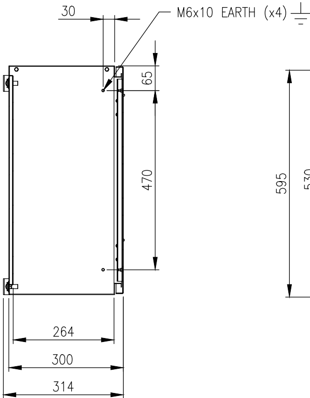
SECTION AY-AY
