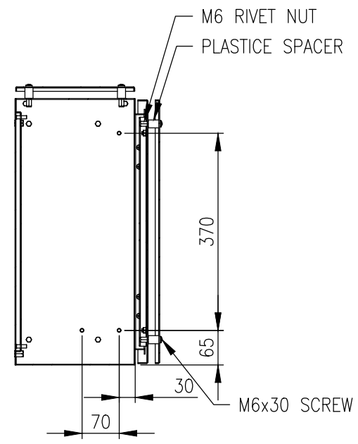
SECTION AV-AV
