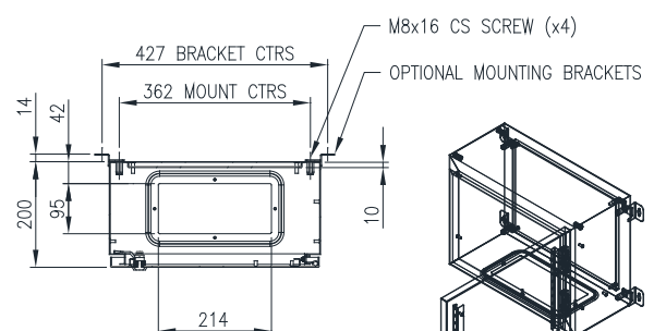
SECTION AV-AV
