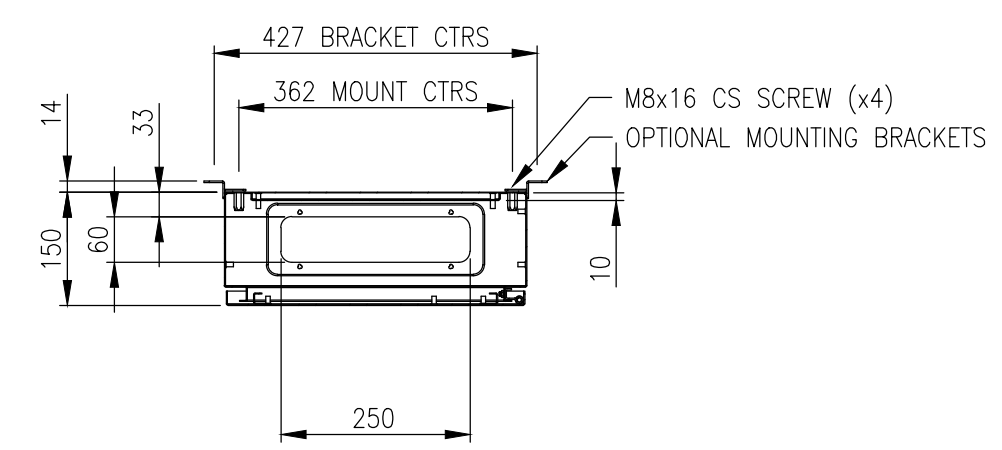
SECTION AV-AV
