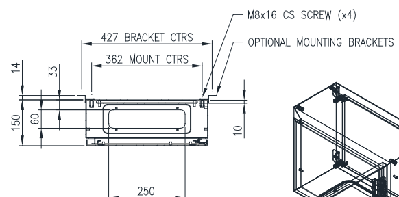
SECTION AV-AV
