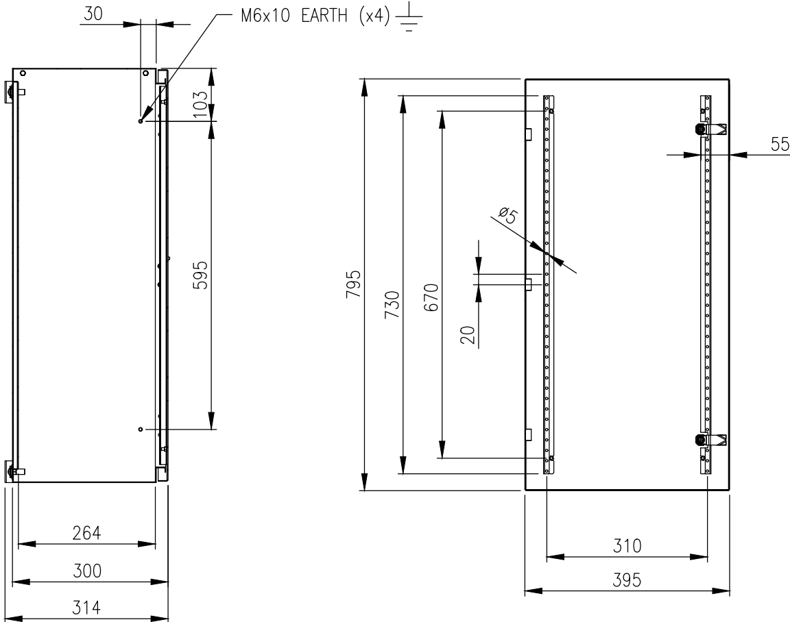
SECTION AY-AY
