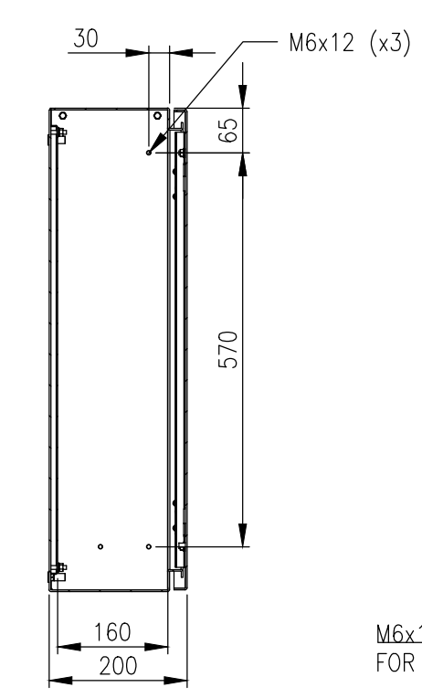
SECTION AY-AY
