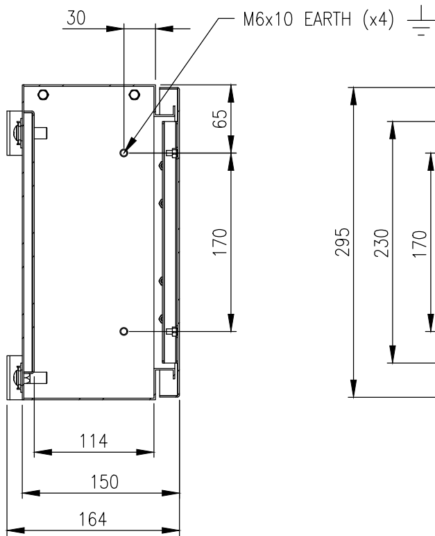
SECTION AV-AV
