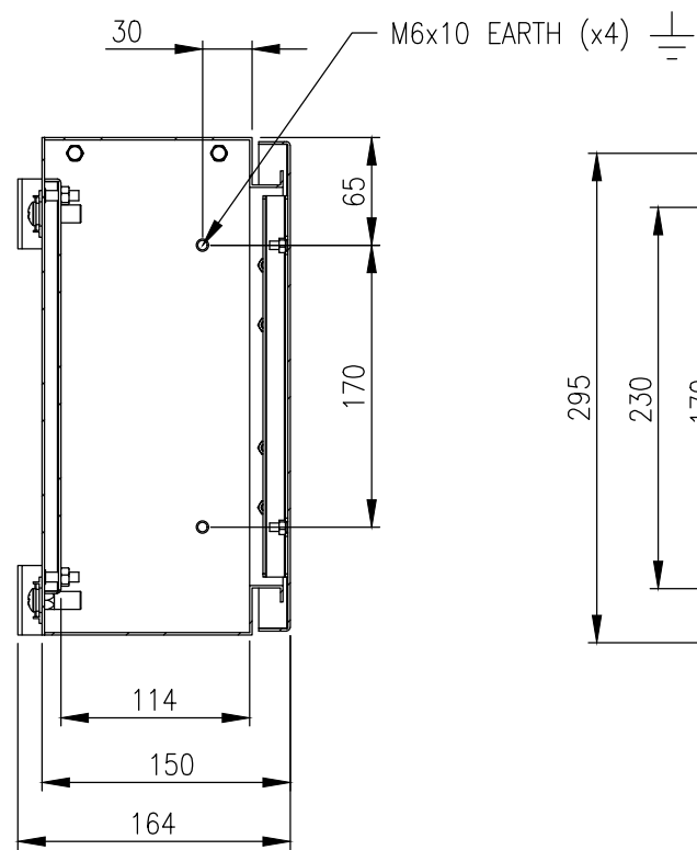
SECTION AV-AV
