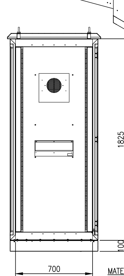
SECTION A-A
