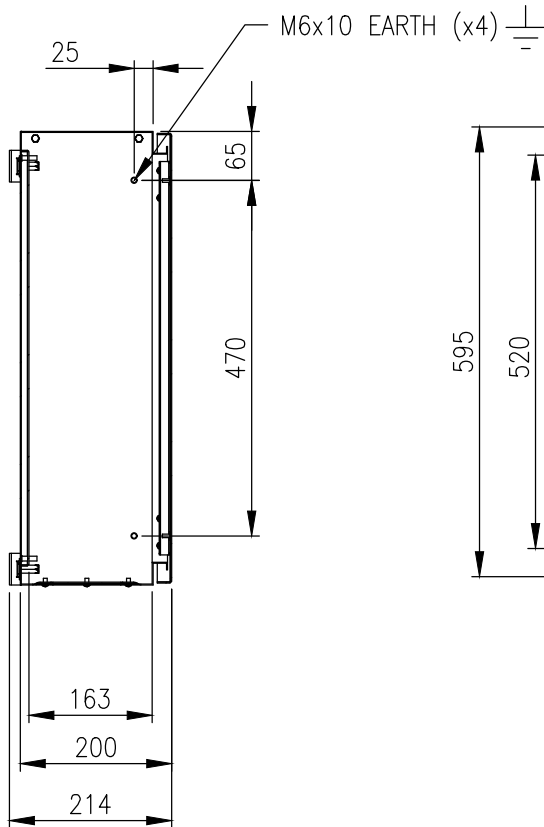
SECTION AV-AV
