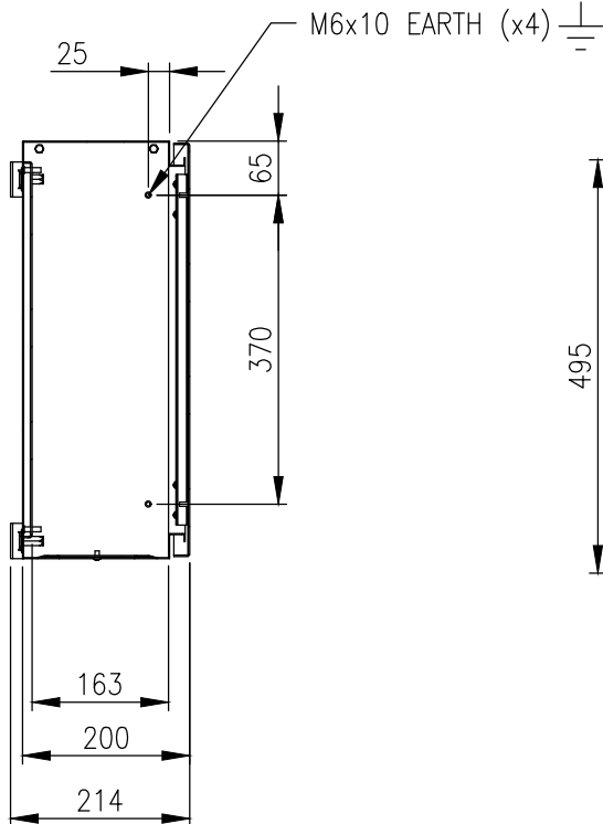
SECTION AV-AV
