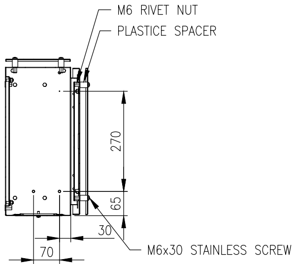
SECTION AV-AV
