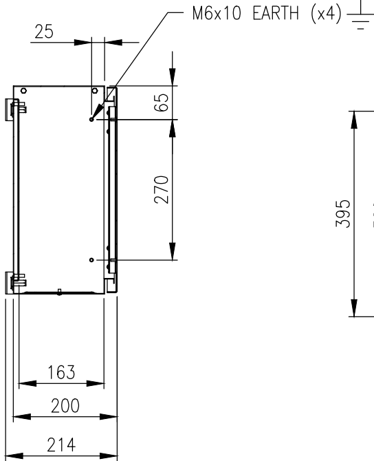
SECTION AV-AV
