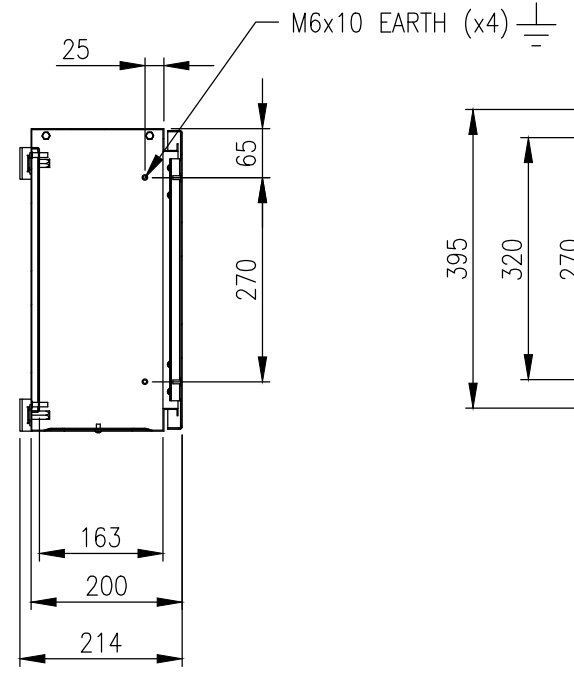
SECTION AV-AV
