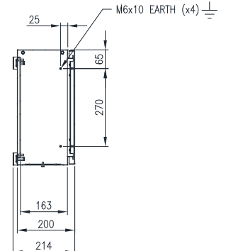
SECTION AV-AV
