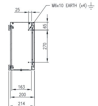
SECTION AV-AV
