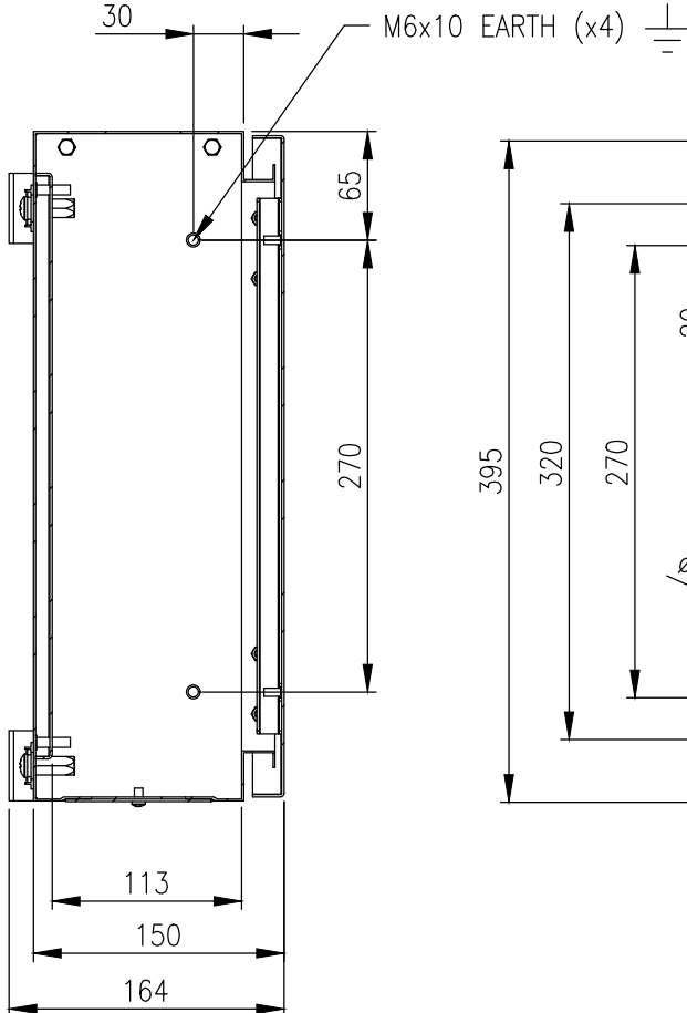
SECTION AV-AV
