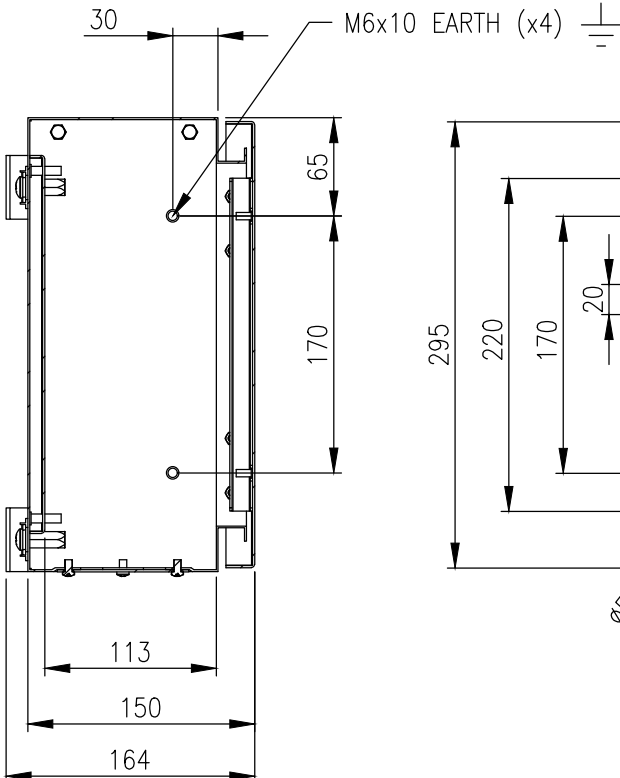
SECTION AV-AV
