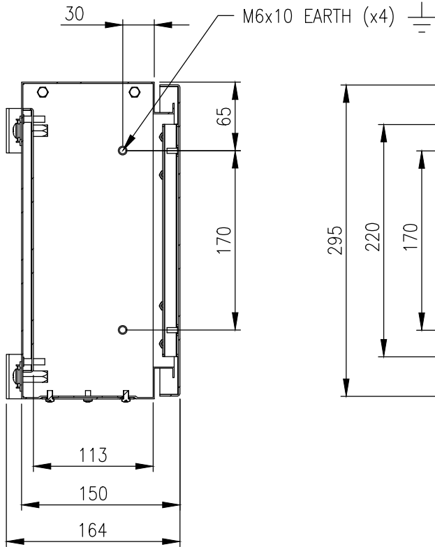
SECTION AV-AV
