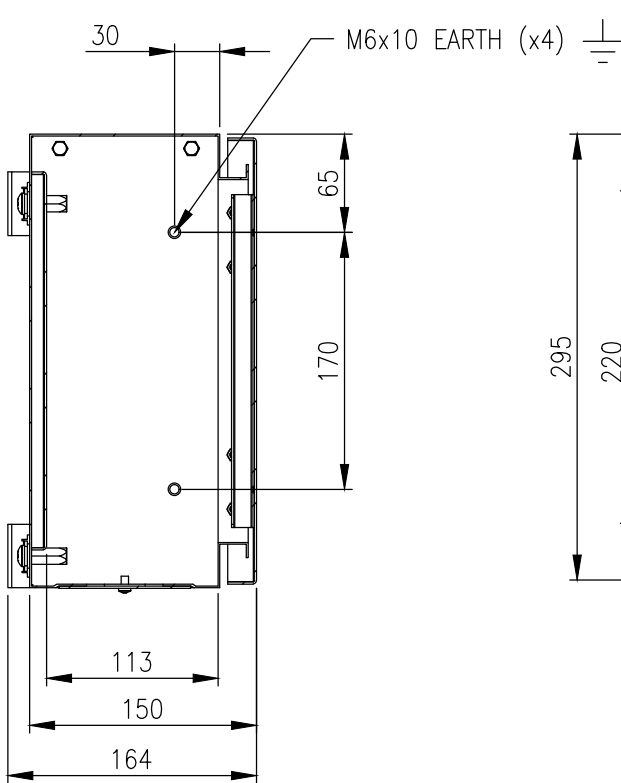
SECTION AV-AV
