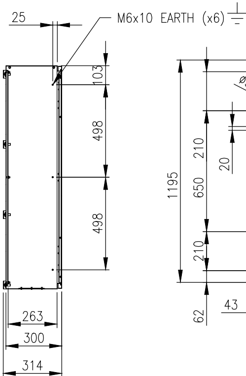
SECTION AV-AV
