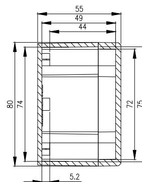
SECTION A-A
